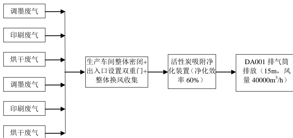
图 4-1 项目废气处理流程图
