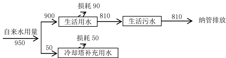
图 2-1 本项目水平衡图（单位：t/a）
