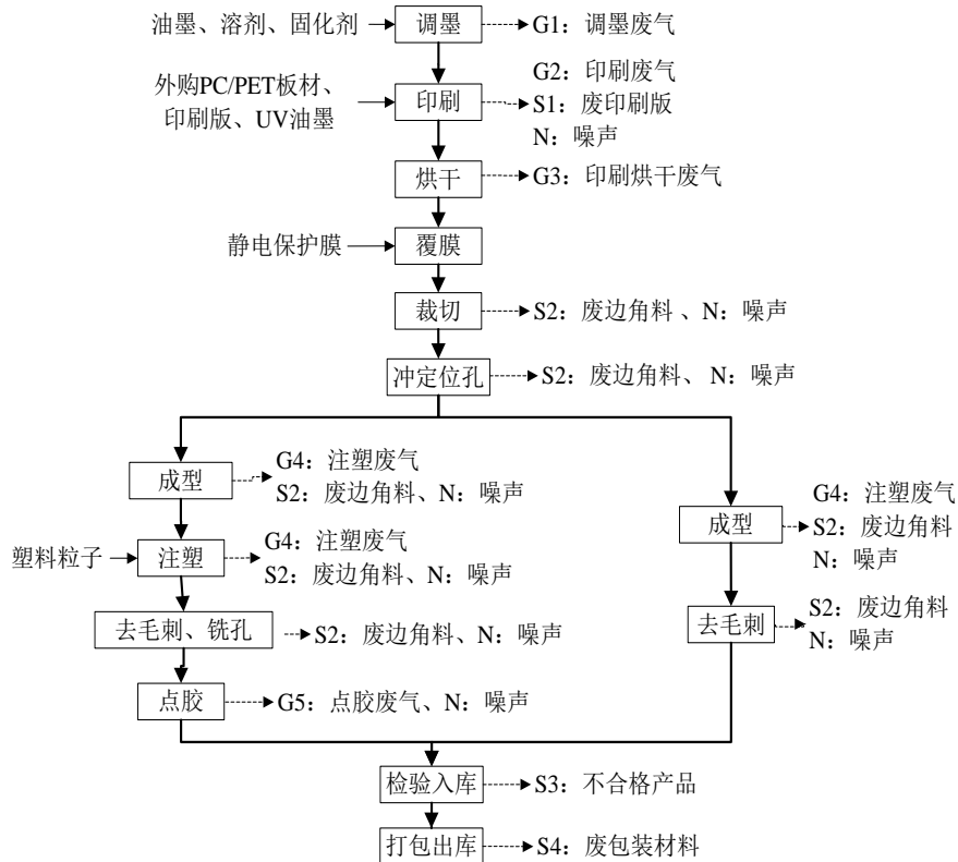
图 2-2 汽车内外饰件生产工艺流程及产污节点图
