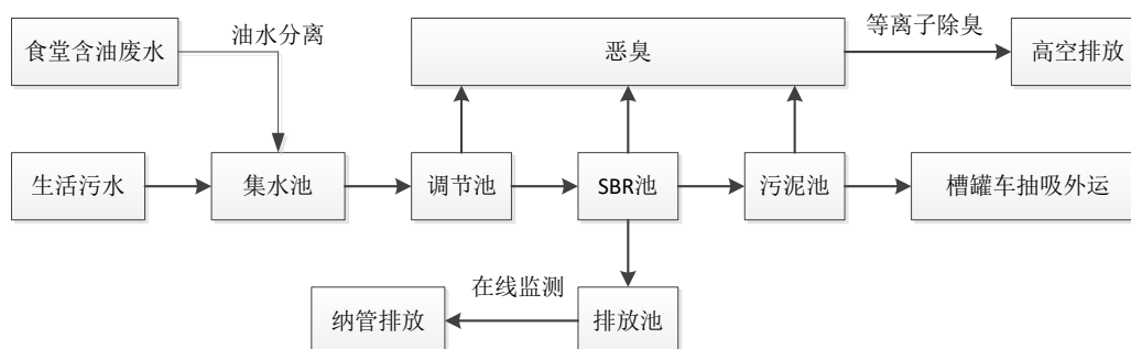
图 3.3.2-4 生活污水处理工艺流程图
