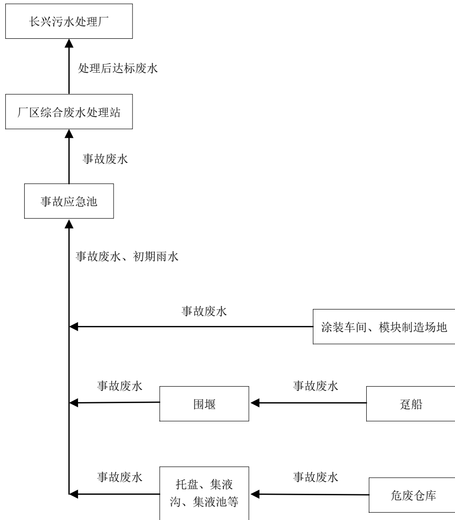
图 7.7.3-1 事故废水控制系统图
