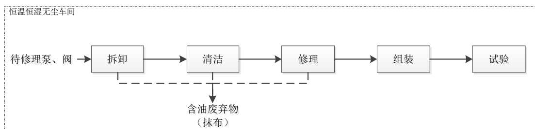
图 3.3.1-9 恒温恒湿无尘车间工艺流程图
