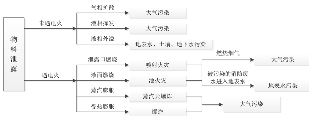
图 3.4.2-1 事故类型及环境影响途径
