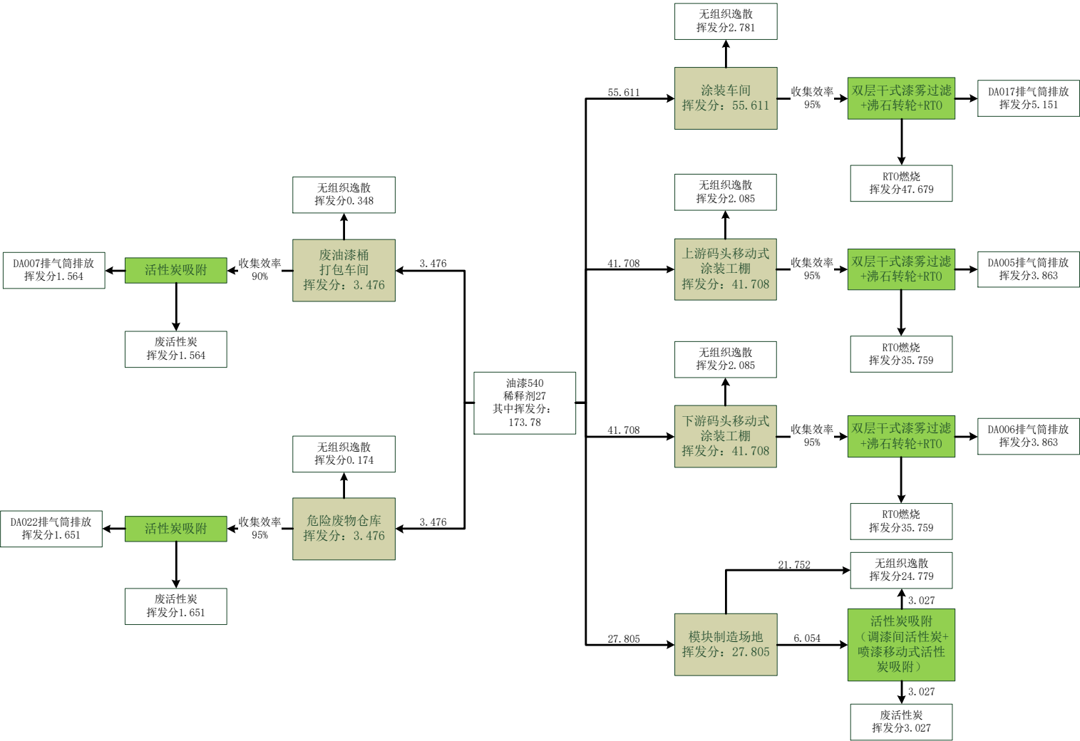
图 4.2.3-5 油漆挥发分平衡（单位 t/a）
