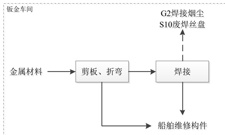
图 3.3.1-8 钣金车间生产工艺流程图
