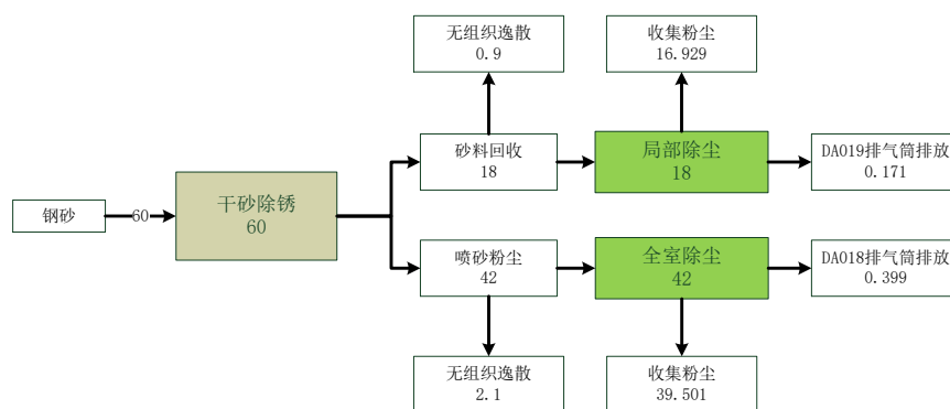
图 4.2.3-7 本工程砂料物料平衡图（单位：t/a）
