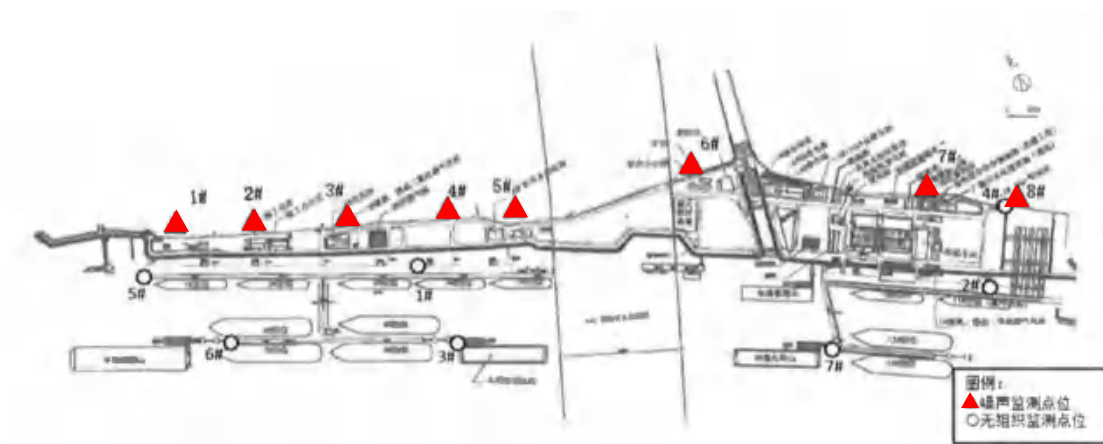
图 3.3.2-7 噪声监测点位图
