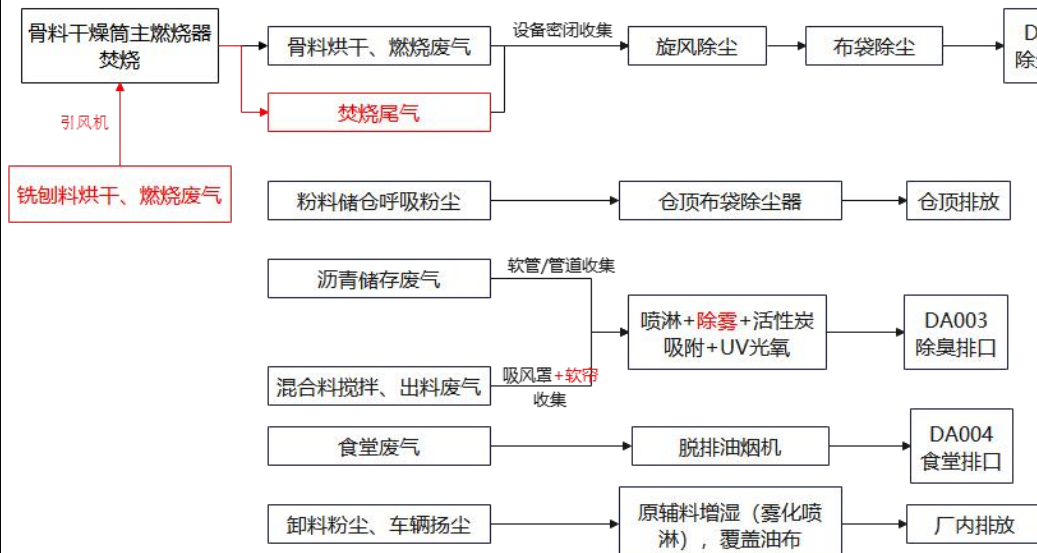
图4-1 本项目建成后全厂废气收集处理系统图
