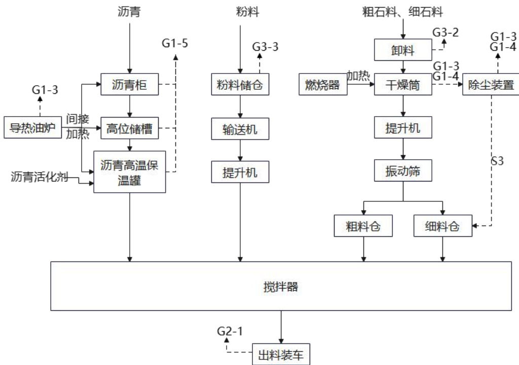
图2-2 现有项目工艺流程图
