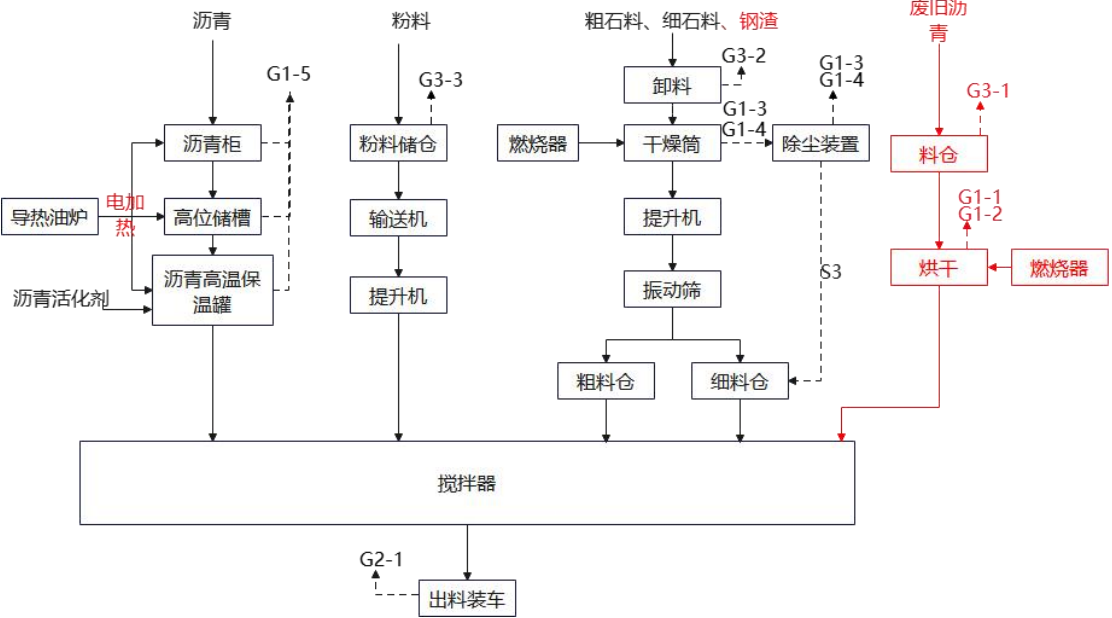
图2-2 本项目建成后全厂工艺流程及产污环节图
