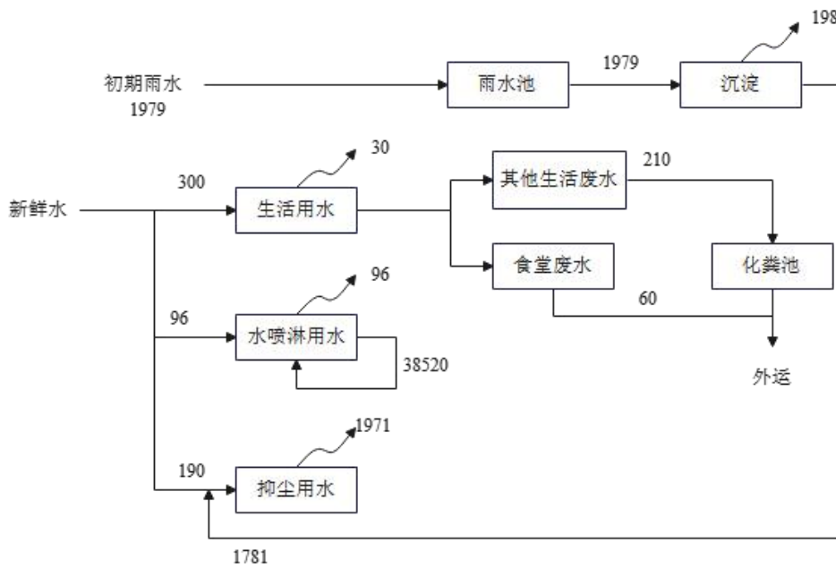
图2-1 本项目实施后全厂水平衡图
