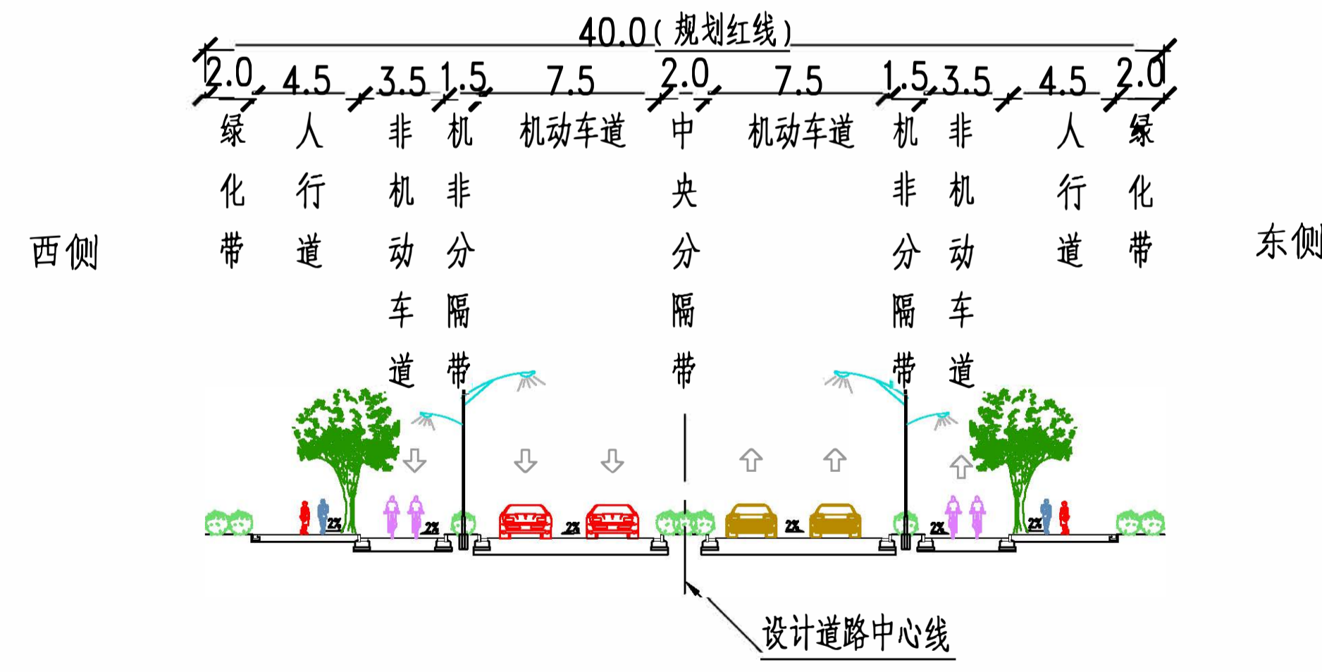
标准横断面设计图
