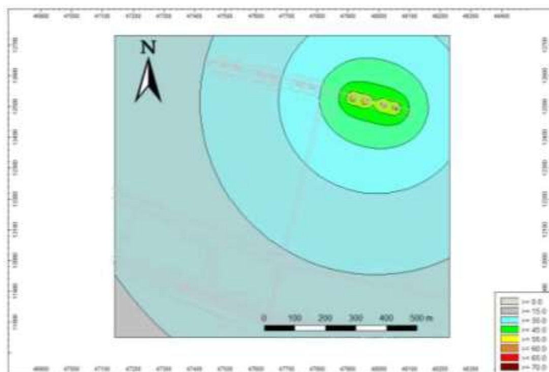
图 7.8-2 噪声预测结果
