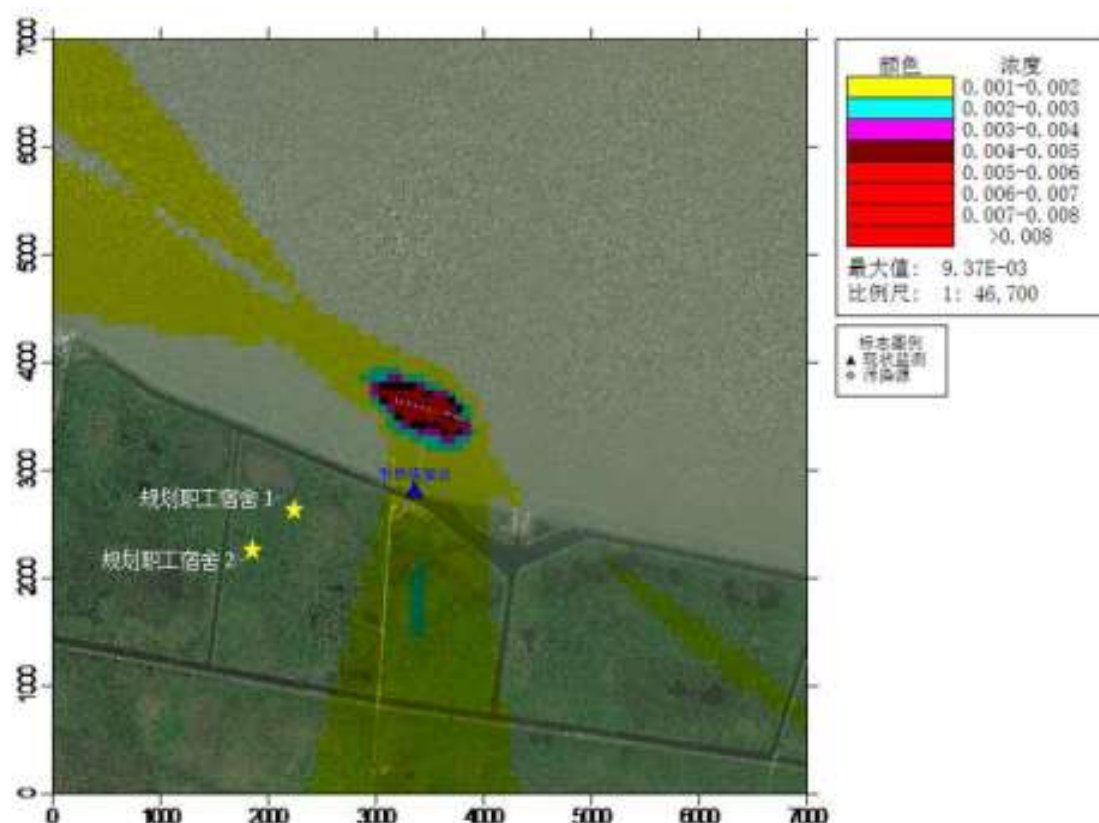
图 7.7-4 PM_{10} 年平均预测浓度（叠加背景值）预测结果图（单位： mg/m^3 ）
