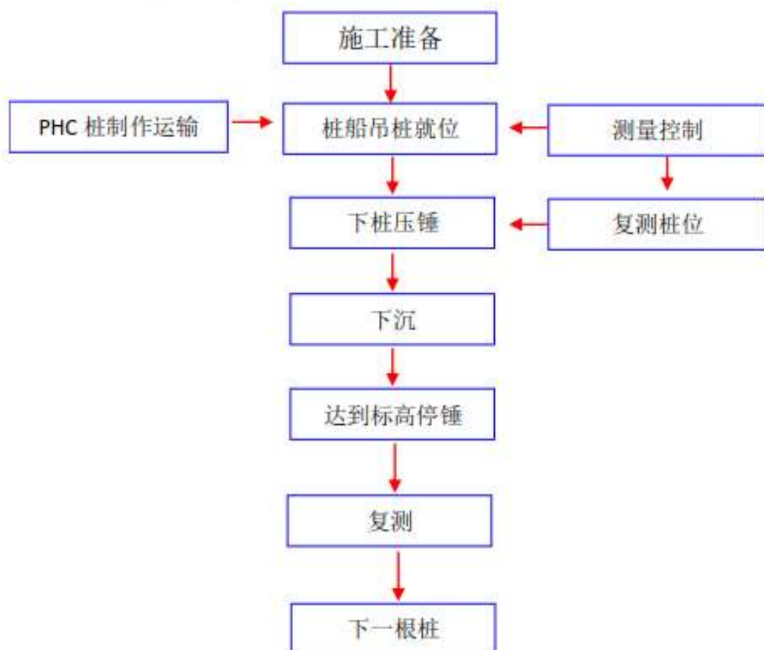
图 4.4-2 沉桩施工工艺流程
