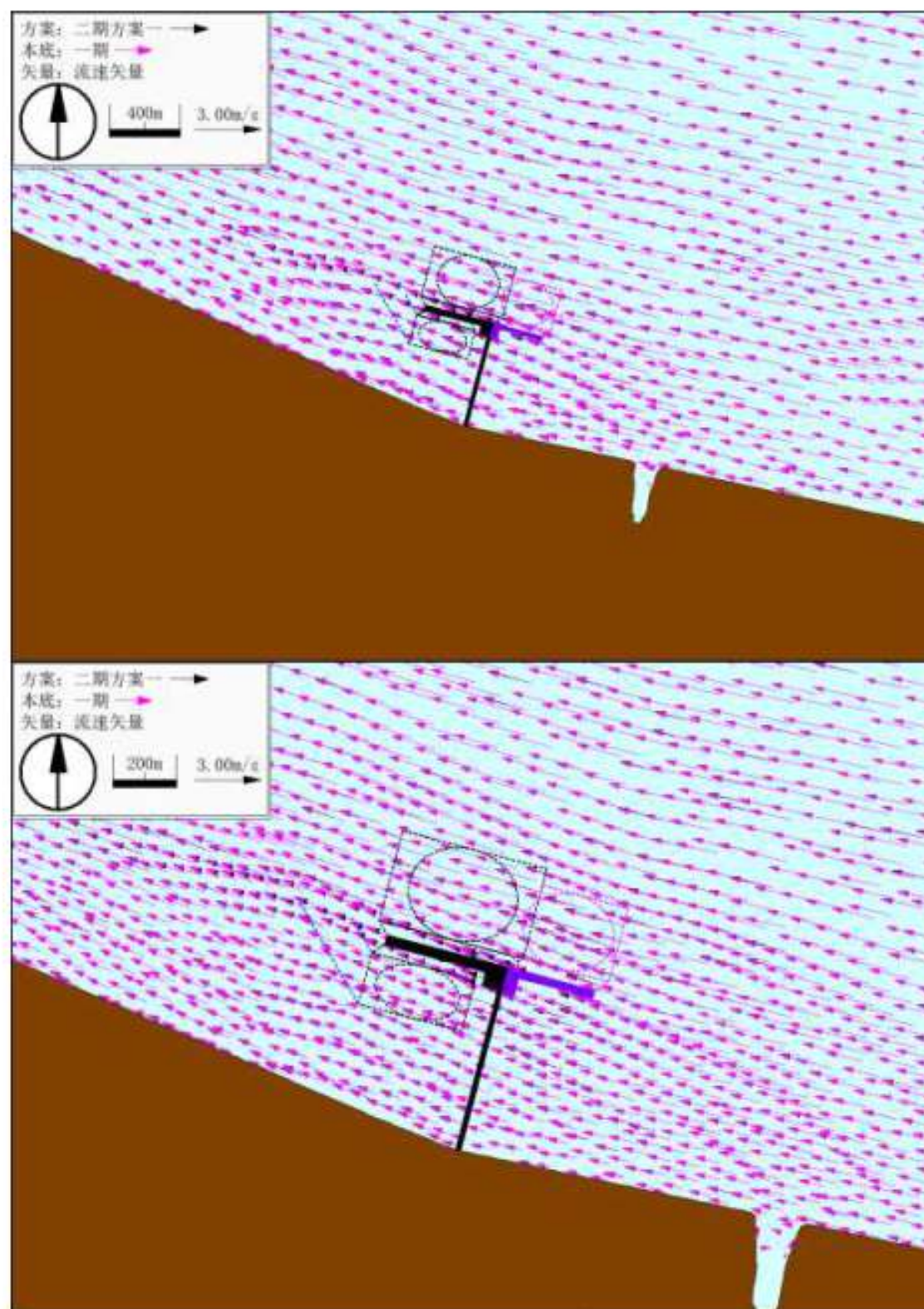
图 7.1-11 工程前后涨急流场 (红线为本底, 黑线为工程后, 下同)
