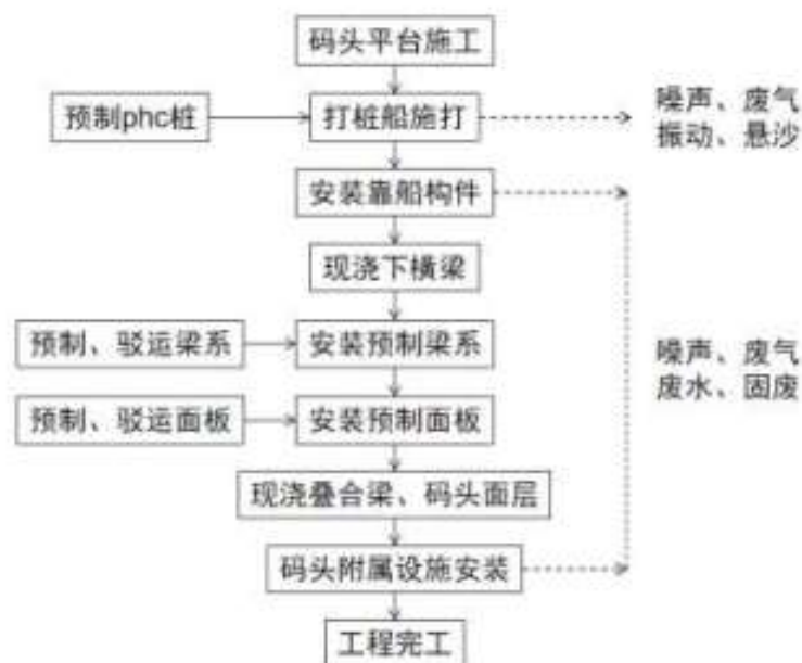
图 5.1-1 码头施工工艺及产污环节图
