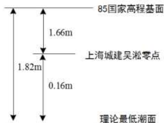
图 6.2-2 共青圩基面关系图
