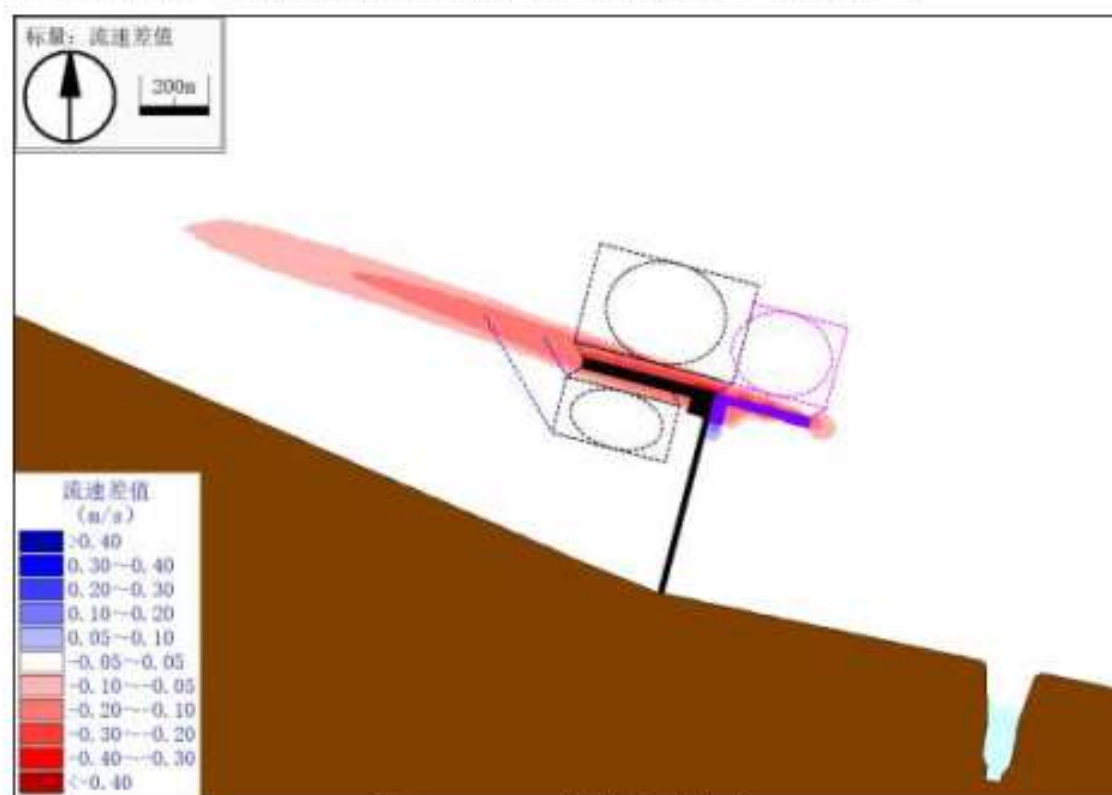
图 7.1-13 涨急流速变化
