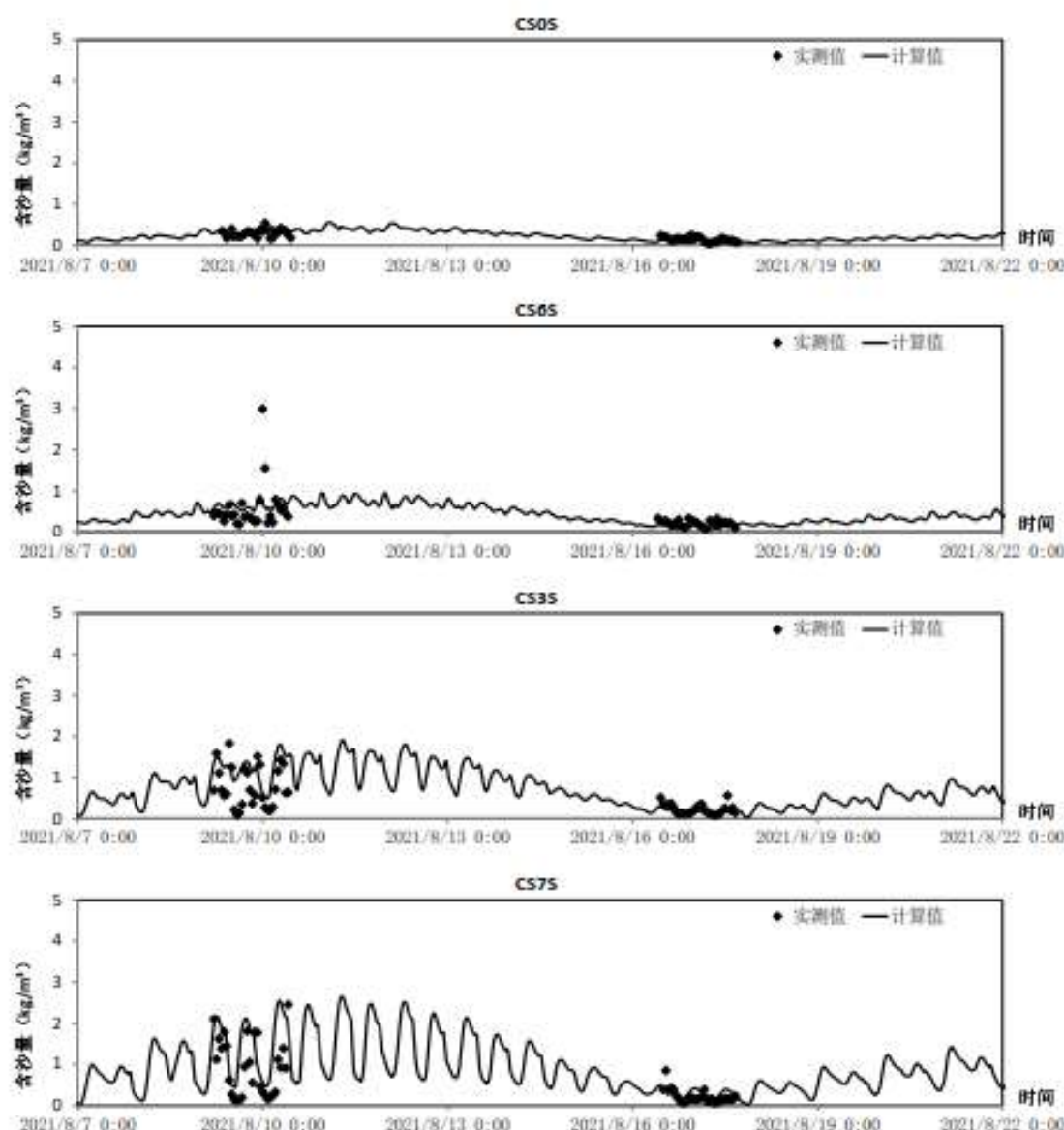
图 7.2-1 含沙量验证图
