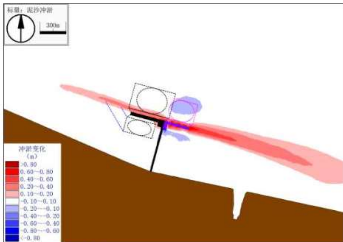
图 7.2-5 工程实施后河床冲淤分布（正为淤积）
