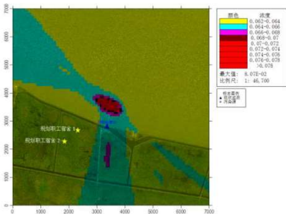
图 7.7-2 TSP 年平均预测浓度 (叠加背景值) 预测结果图 (单位: \text{mg}/\text{m}^3 )
