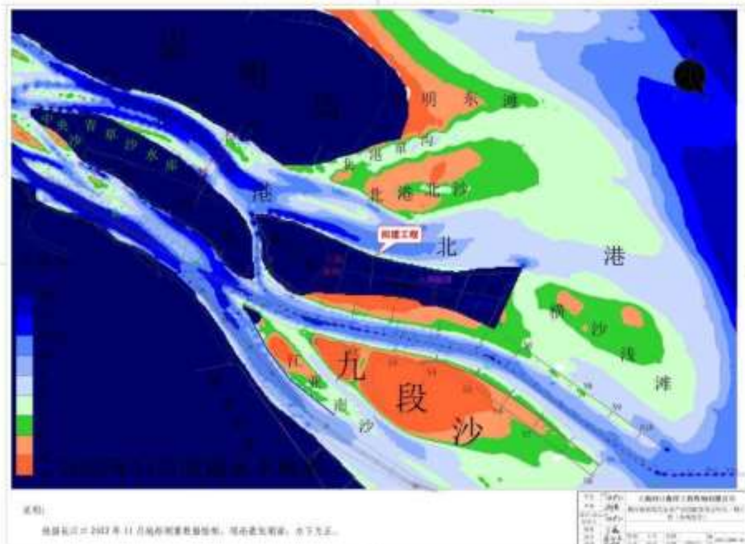
图 6.3-1 长江口北港水下地形图
