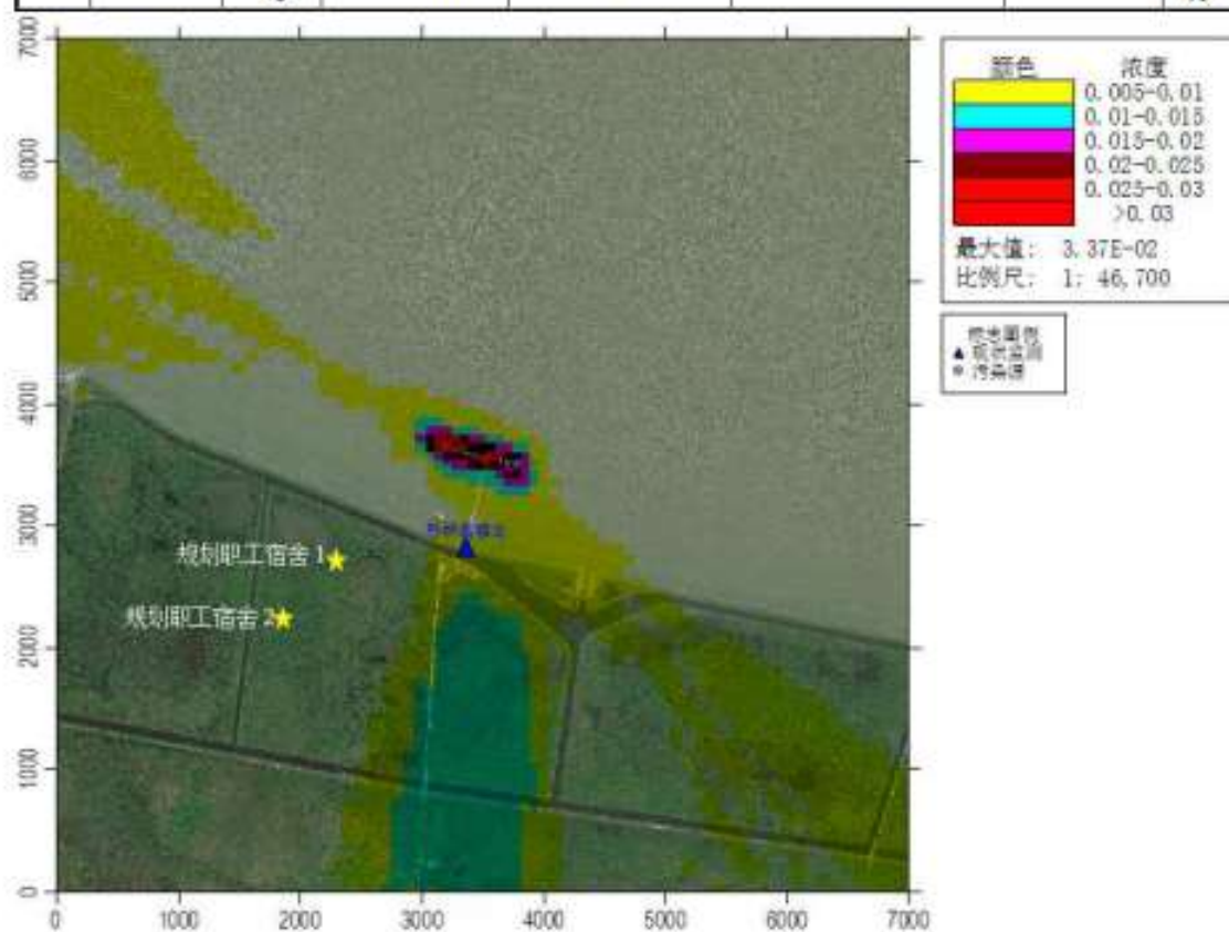
图 7.7-3 \text{PM}_{10} 日平均预测浓度 (叠加背景值) 预测结果图 (单位: \text{mg}/\text{m}^3 )
