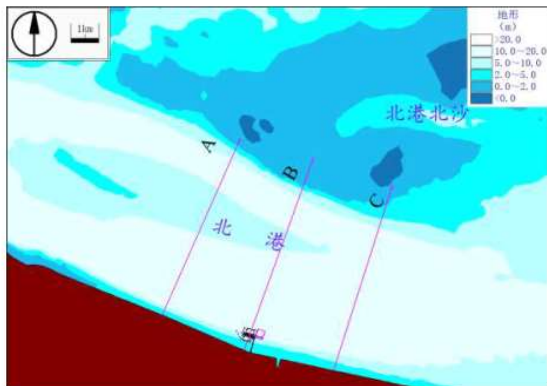
图 7.1-16 潮通量断面位置示意图
