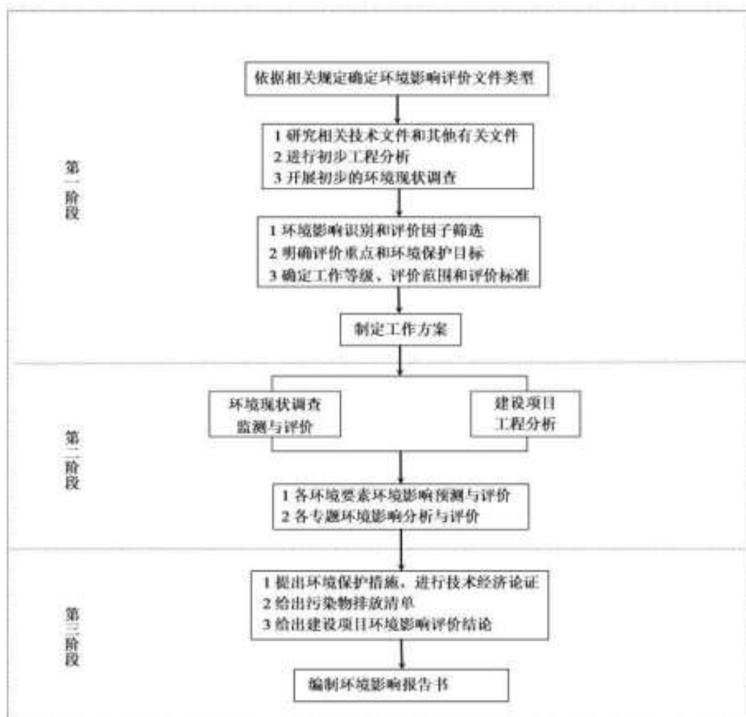
图 2.8-1 本工程环境影响评价工作技术路线图
