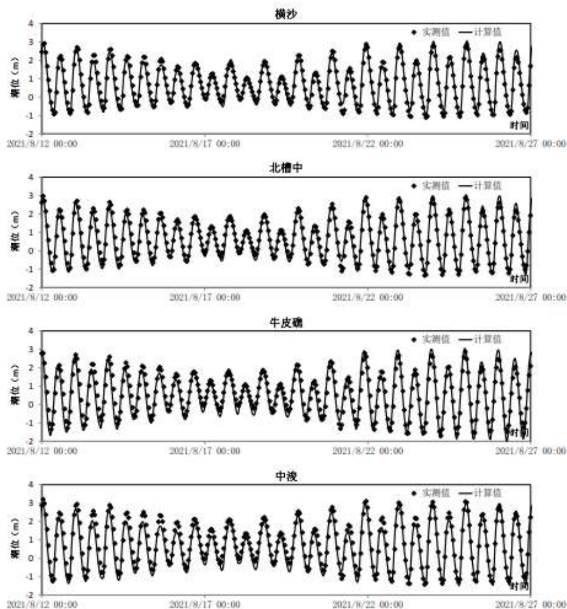
图 7.1-5 潮位验证图
