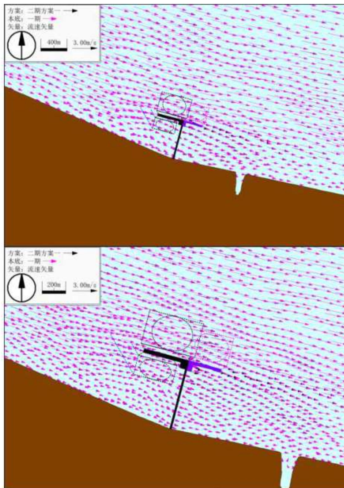
图 7.1-12 工程前后落急流场
