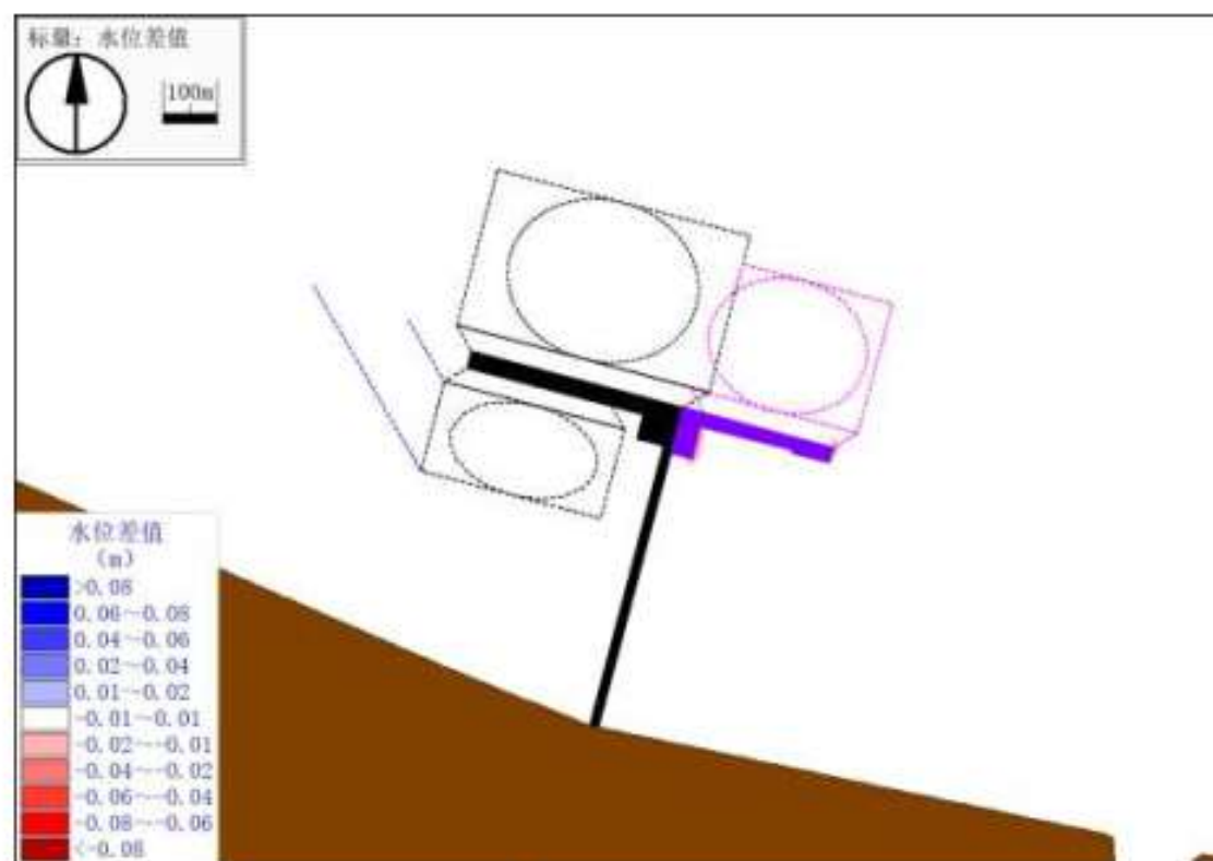
图 7.1-10 大潮低潮位变化
