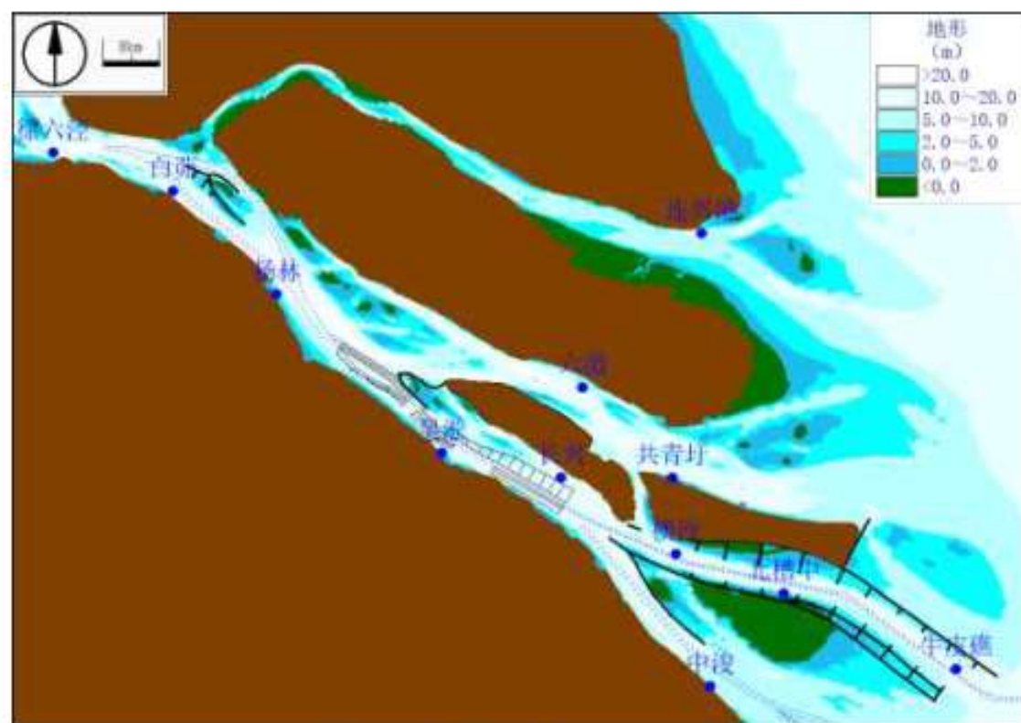
图 7.1-3 2021 年 8 月潮位站位置图
