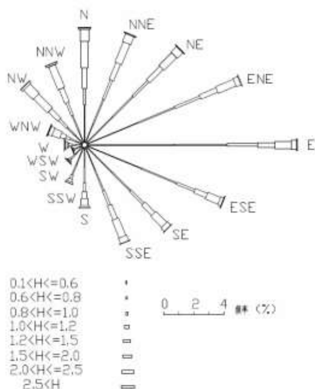
图 6.1-3 引水船站波浪玫瑰图
