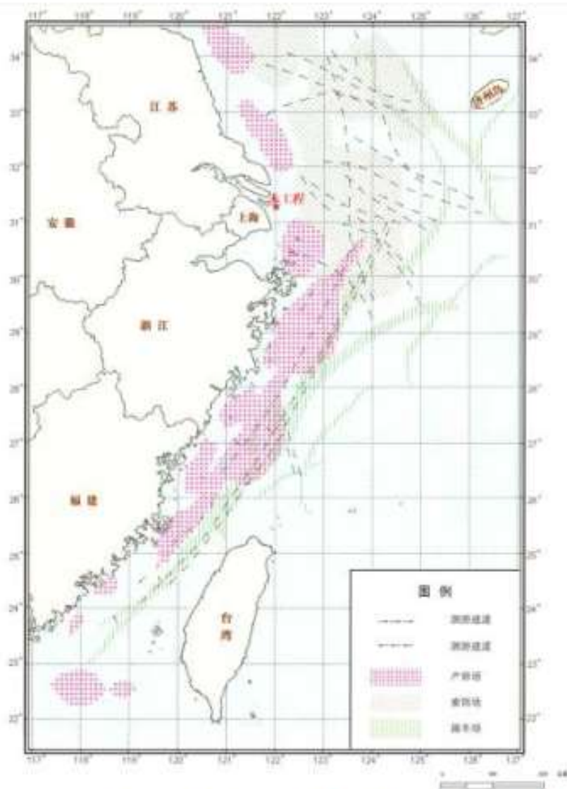
图 6.10-6 东海近海中上层鱼类分布洄游示意图
