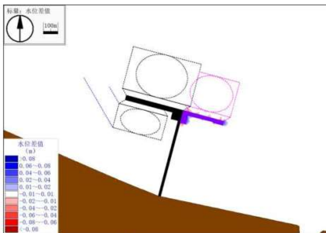
图 7.1-9 大潮高潮位变化
