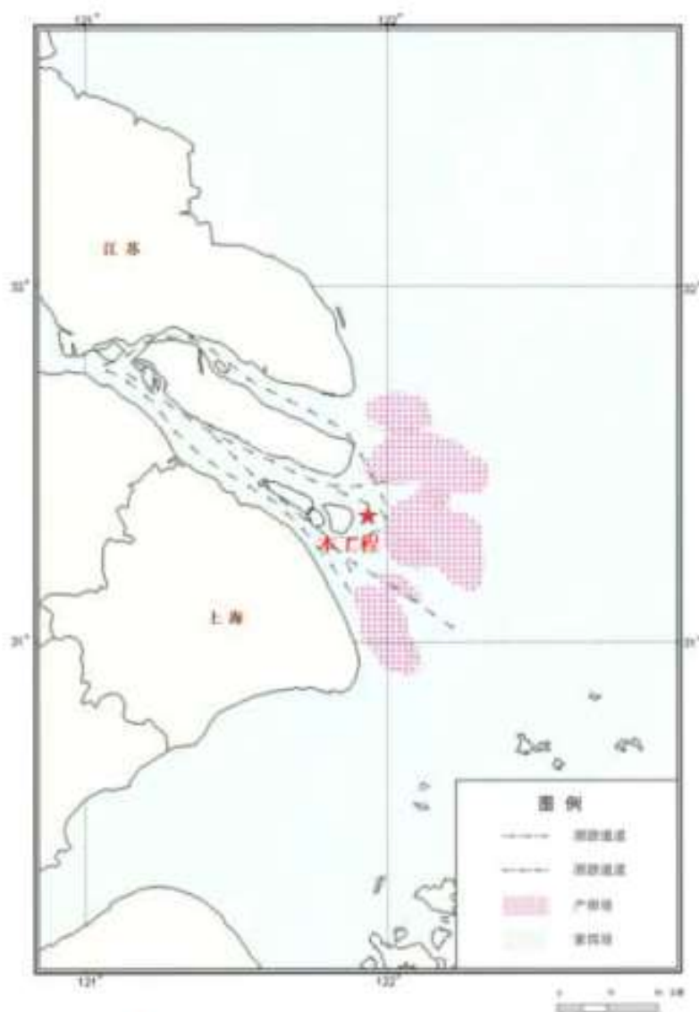
图 6.10-4 东海长江口虾蟹类分布洄游示意图
