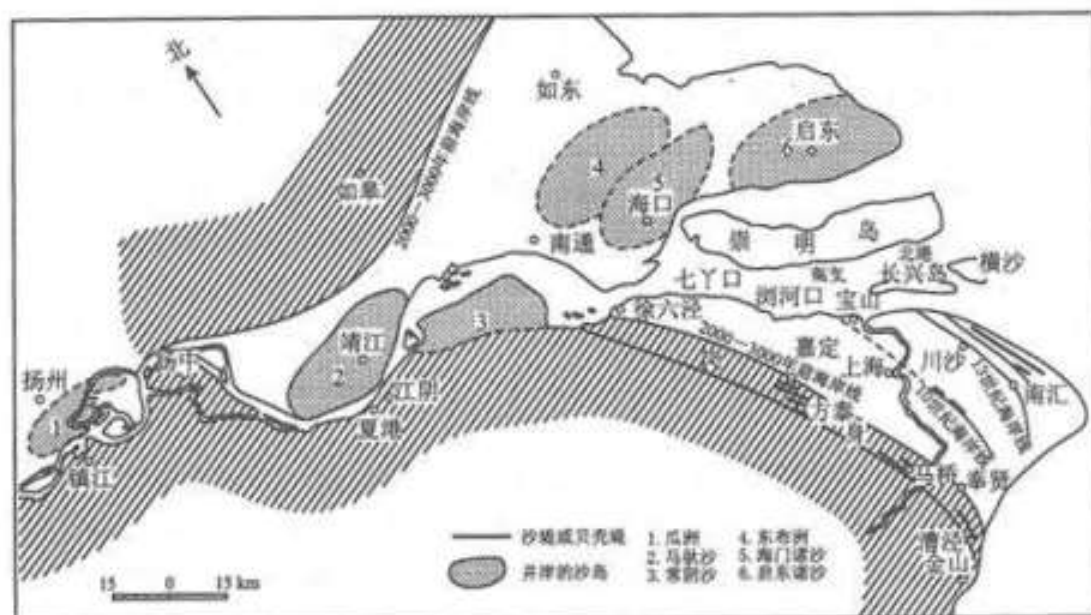
图 6.3-19 长江河口历史变迁
