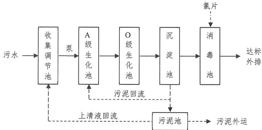
图3 废水处理装置工艺流程图
