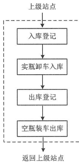
图1 本项目钢瓶贮存流程及产污节点图
