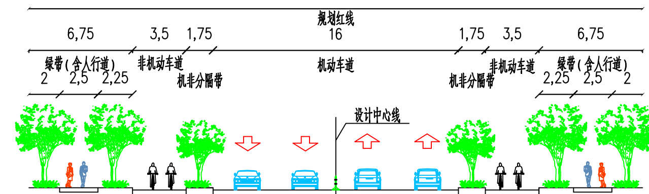
道路标准横断面设计面
