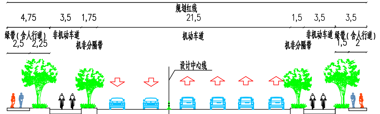
道路交叉口渠化段横断面设计面
